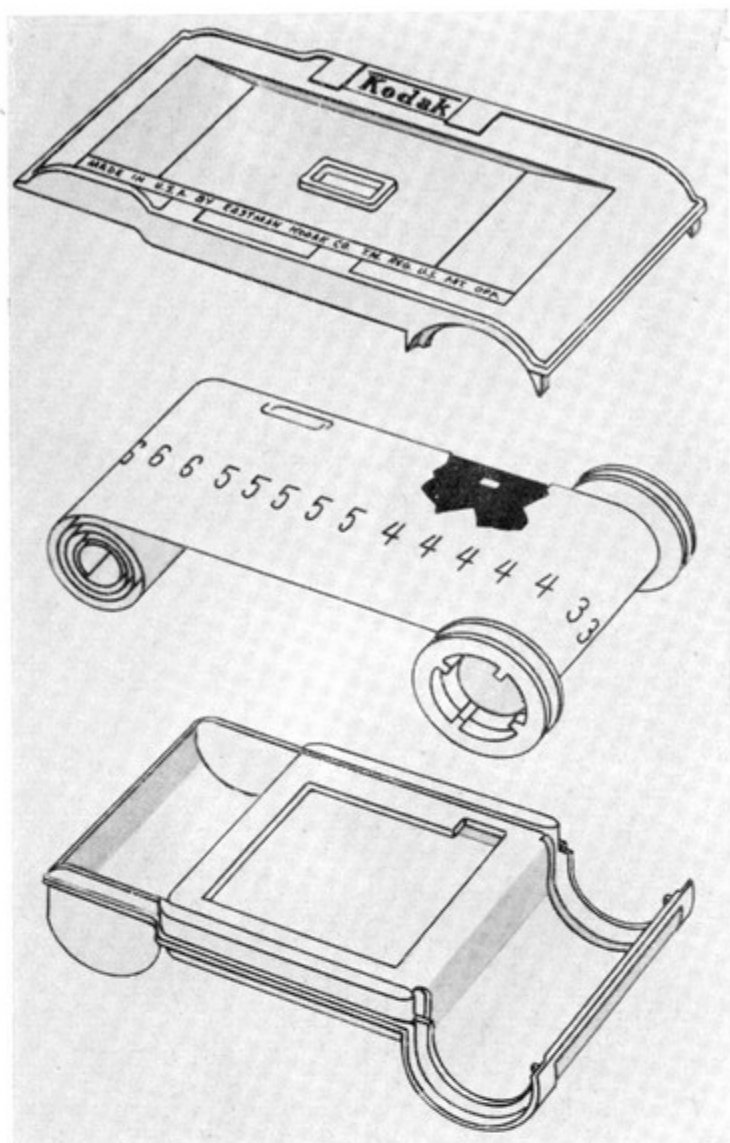
Il «Kodapak» nelle sue tre parti: in quella superiore si vede la finestrina per la numerazione, e nella centrale il foro nella pellicola tra una negativa e l'altra per l'arresto automatico.
